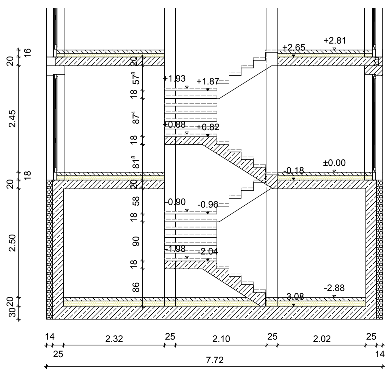
Treppenschnitt D-D (KG - OG)
